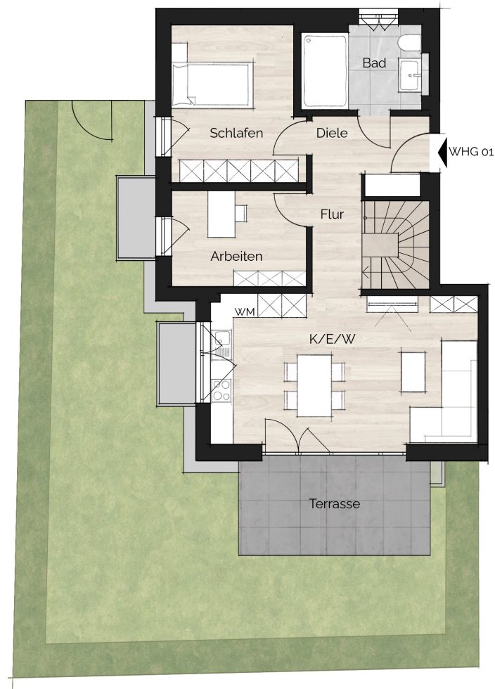
Wohnung 1 EG
